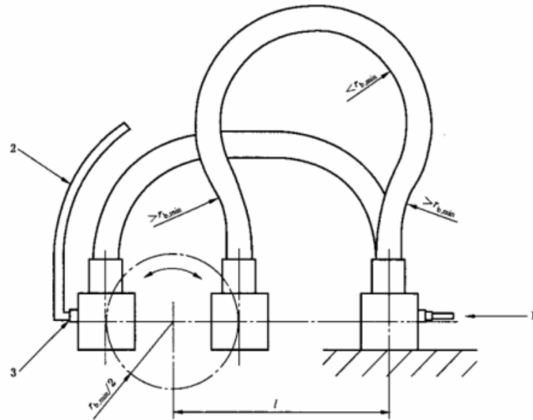
图例： 1——试验压力入口； 2——流体循环管； 3——止回阀。
